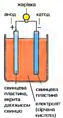
Акумулятор електричний Схематична будова свинцевого акумулятора
